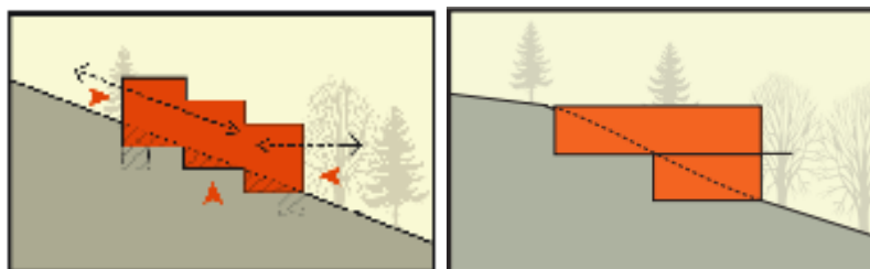
Illustration de la règle : réduire les terrassements en s'adaptant à la pente
